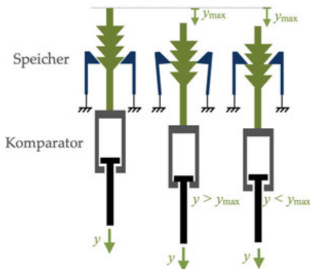
Bild 7 Maximalwertspeicher
