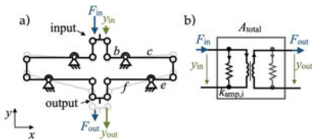
Bild 6 a) Mechanischer Transformator und b) Vierpol-Ersatzschaltbild
