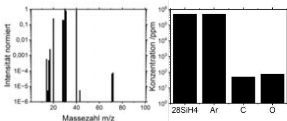
Bild 2 Gas-MS-Spektren der ^{28}\text{SiH}_4 -Proben.
