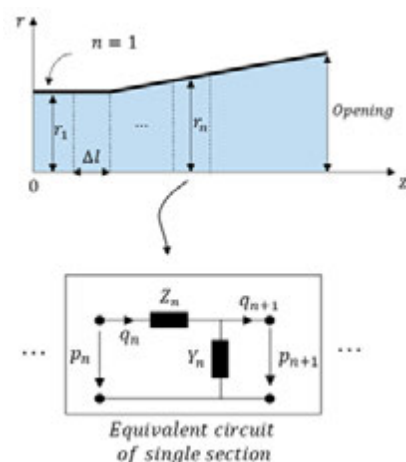
Bild 4 Modellierung des akustischen Horns, mittels eines diskretisierten akustischen Transmissionline-Modells.
