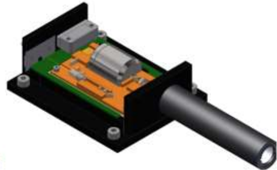
Bild 4 Renderbild der mechanischen Zeichnung des Quanteninterferenzmoduls.
