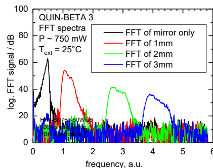
Bild 10 Fast Furier Transformierte (FFT) der QI-Spektren aus denen sich, bei bekanntem Brechungsindex, direkt die Dicke der Proben ableiten lässt.
